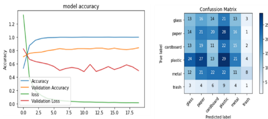
Figura 3. Métricas de entrenamiento modelo VGG-16
