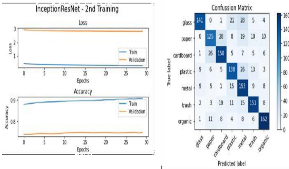
Figura 5. Métricas segundo entrenamiento modelo InceptionResNet
