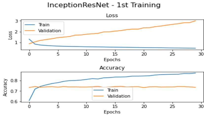
Figura 4. Métricas primer entrenamiento modelo InceptionResNet
