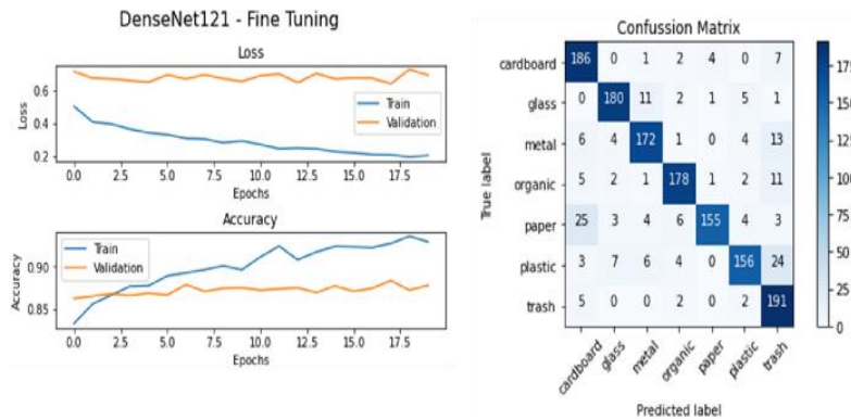
Figura 2. Métricas segundo entrenamiento modelo DenseNet121
