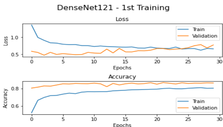
Figura 1. Métricas primer entrenamiento modelo DenseNet121
